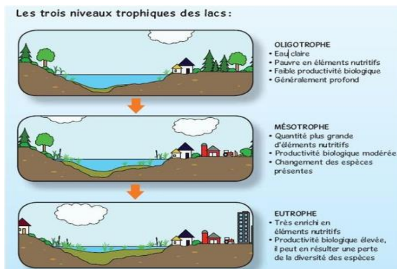
Figure 39 : les différents états trophique d'un lac (federationdeslacs.ca)
