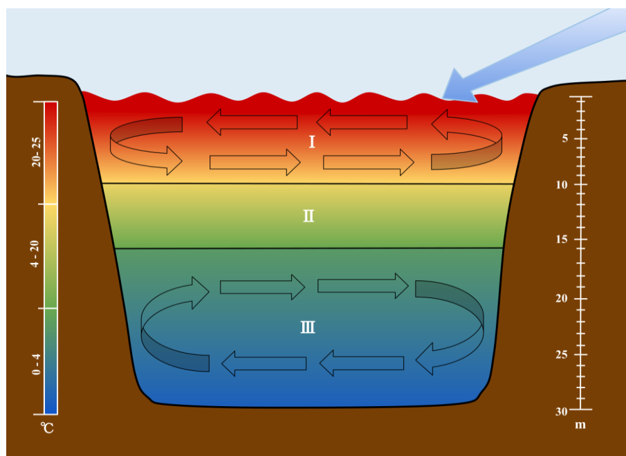
Figure 37 : Couches de stratification thermique d'un lac (aquaportail.com)
