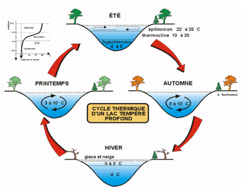
Figure 38 : Dynamique du cycle de stratification annuel d'un lac (lacs-en-danger.chez-alice.fr)
